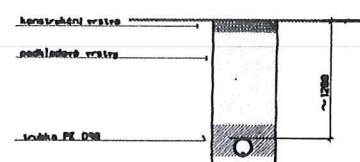
ULOŽENÍ KABELU NN V KOMUNIKACI - PROTĚLAK
