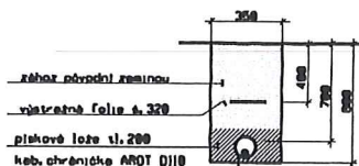
ULOŽENÍ KABELU NN VE VOLNÉM TERÉNU
