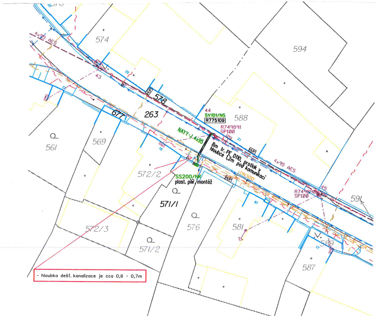
ULOŽENÍ KABELU NN VE VOLNÉM TERÉNU
